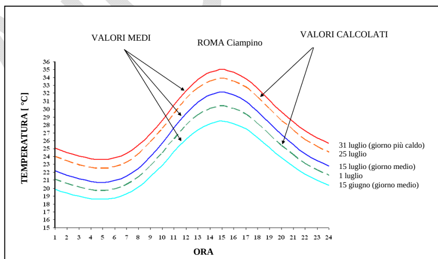
Fig. G.3 - Andamento orario dei valori della temperatura in giorni intermedi
