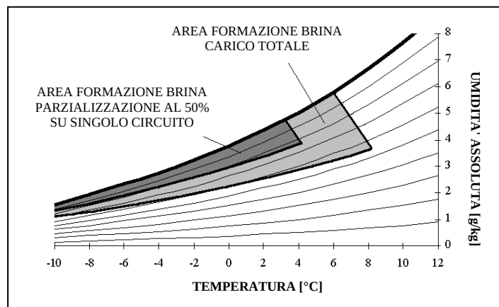
Fig. H.2 - Confronto tra le aree di formazione di brina sulle batterie evaporanti nel caso di pieno carico e in quello di parzializzazione
