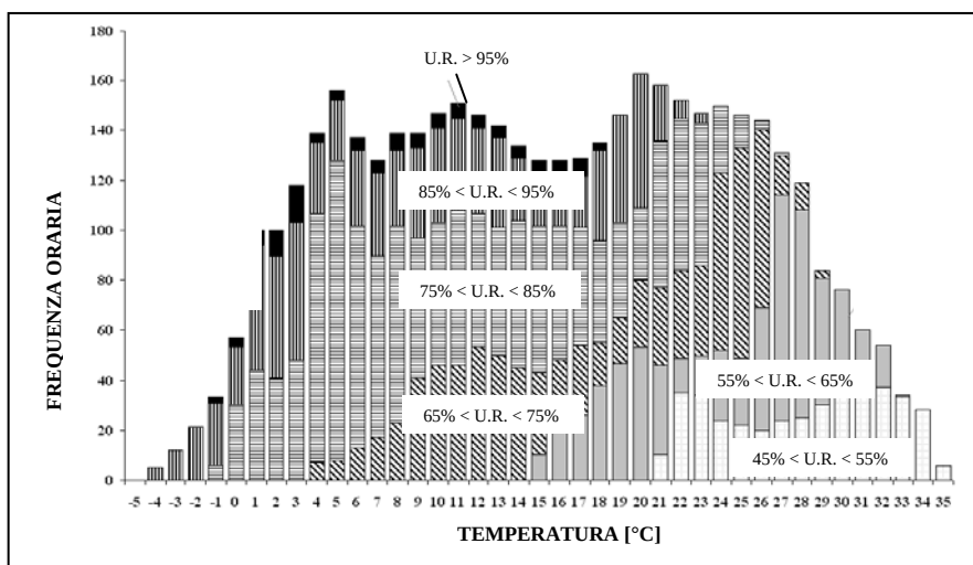
Fig. 2.5 - Superamento del secondo limite del Bin Method: frequenza oraria divisa su più fasce di valori di umidità relativa per una città dell'Italia settentrionale, ore diurne
