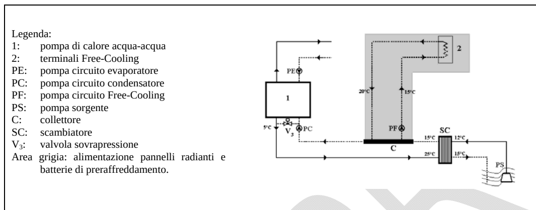
Fig. C.5 - Free-Cooling estivo da sorgente geotermica
