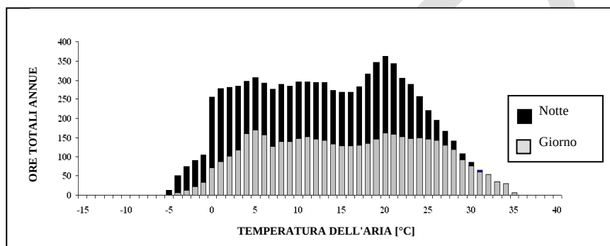
Fig. 2.3 - Superamento del primo limite del Bin Method: costruzione di curve di frequenza oraria differenziate per giorno e notte in riferimento a una città dell' Italia settentrionale
