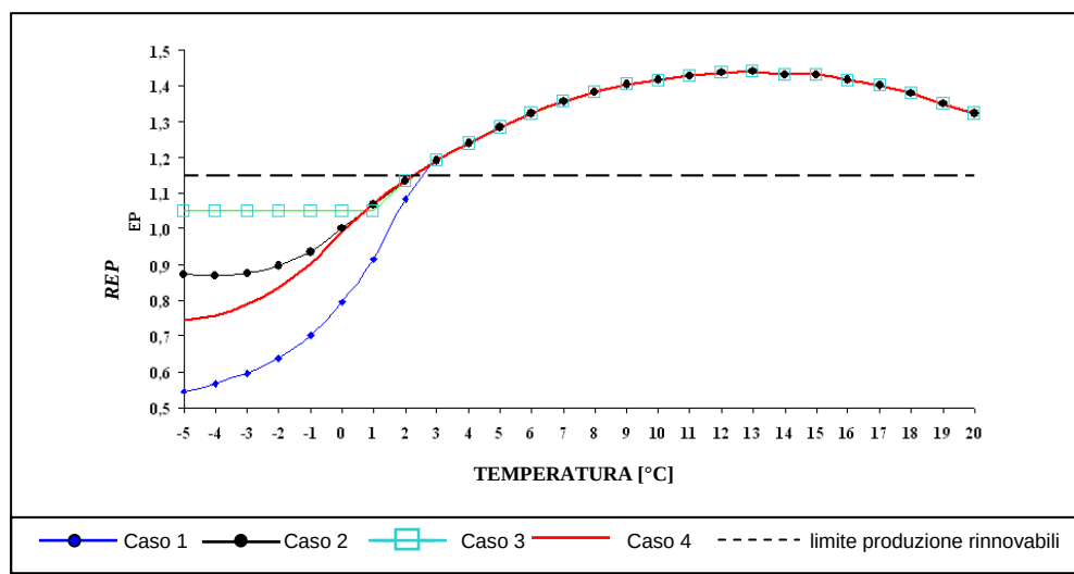
Fig. 1.5 - REp di sistema misto in funzione dei valori della temperatura dell'aria esterna
