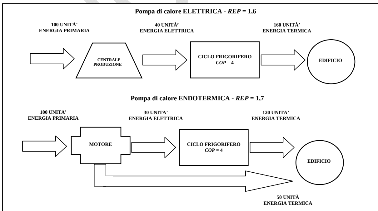
Fig. 1.3 - Bilancio di energia su pompe di calore con compressore elettrico e con compressore calettato a un motore endotermico. Il COP del ciclo frigorifero è uguale in entrambi i casi
