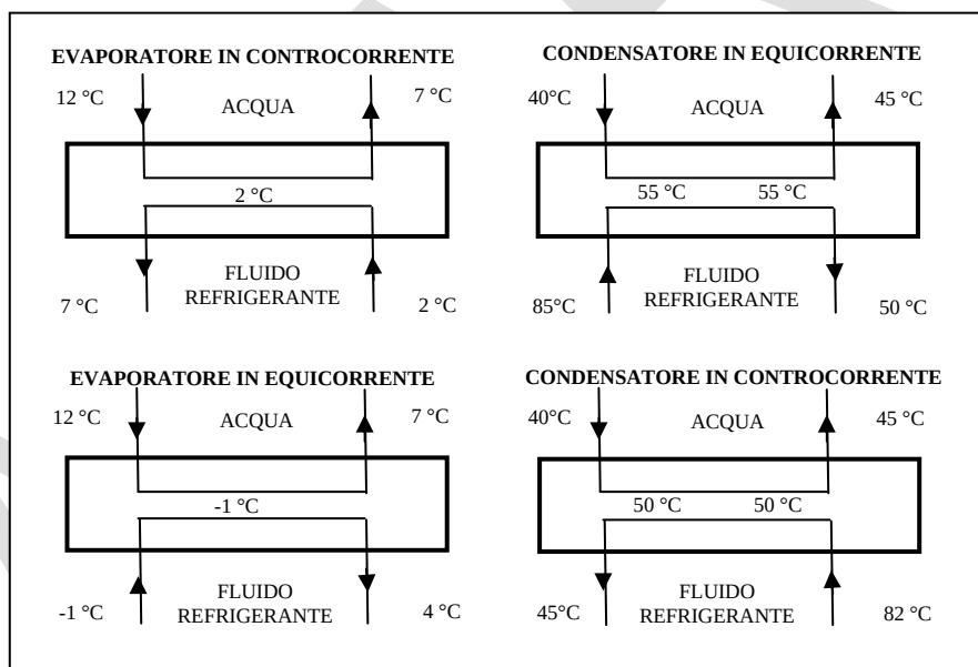
Fig. F.1 - Inversione del fluido refrigerante negli scambiatori in pompe di calore a inversione sul ciclo frigorifero
